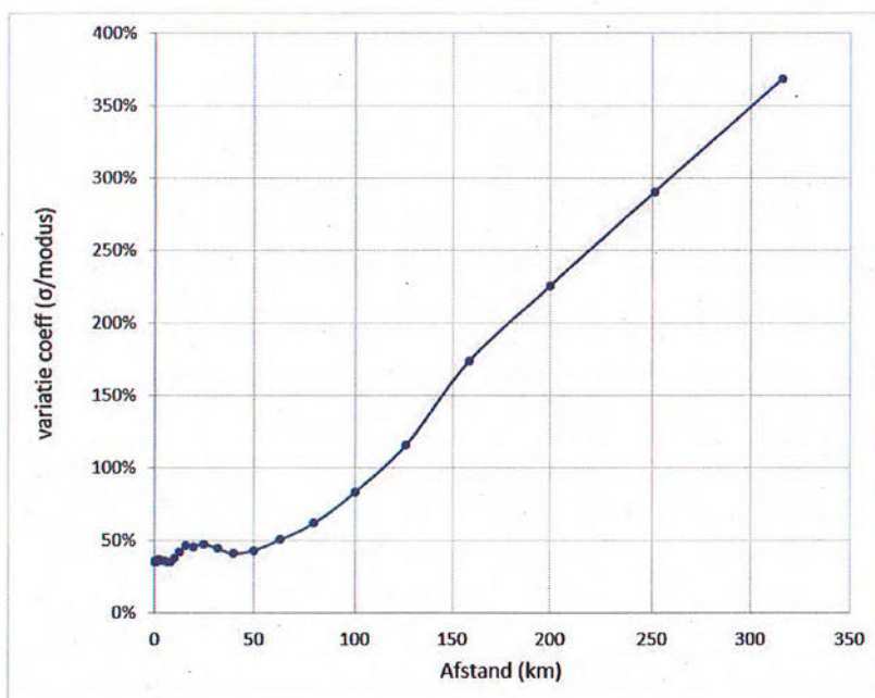
Figuur 4 De variatiecoëfficiënt in de depositie van ammoniak zoals berekend in Figuur 3. (Weergegeven is de standaarddeviatie ( \sigma ) gedeeld door de depositie) als functie van de afstand tot die stal bij willekeurige variatie van de depositiesnelheid ( v_d ), de hoogte van de menglaag, de windrichting, de oppervlakteruwheid en de achtergrondconcentratie van ammoniak.
